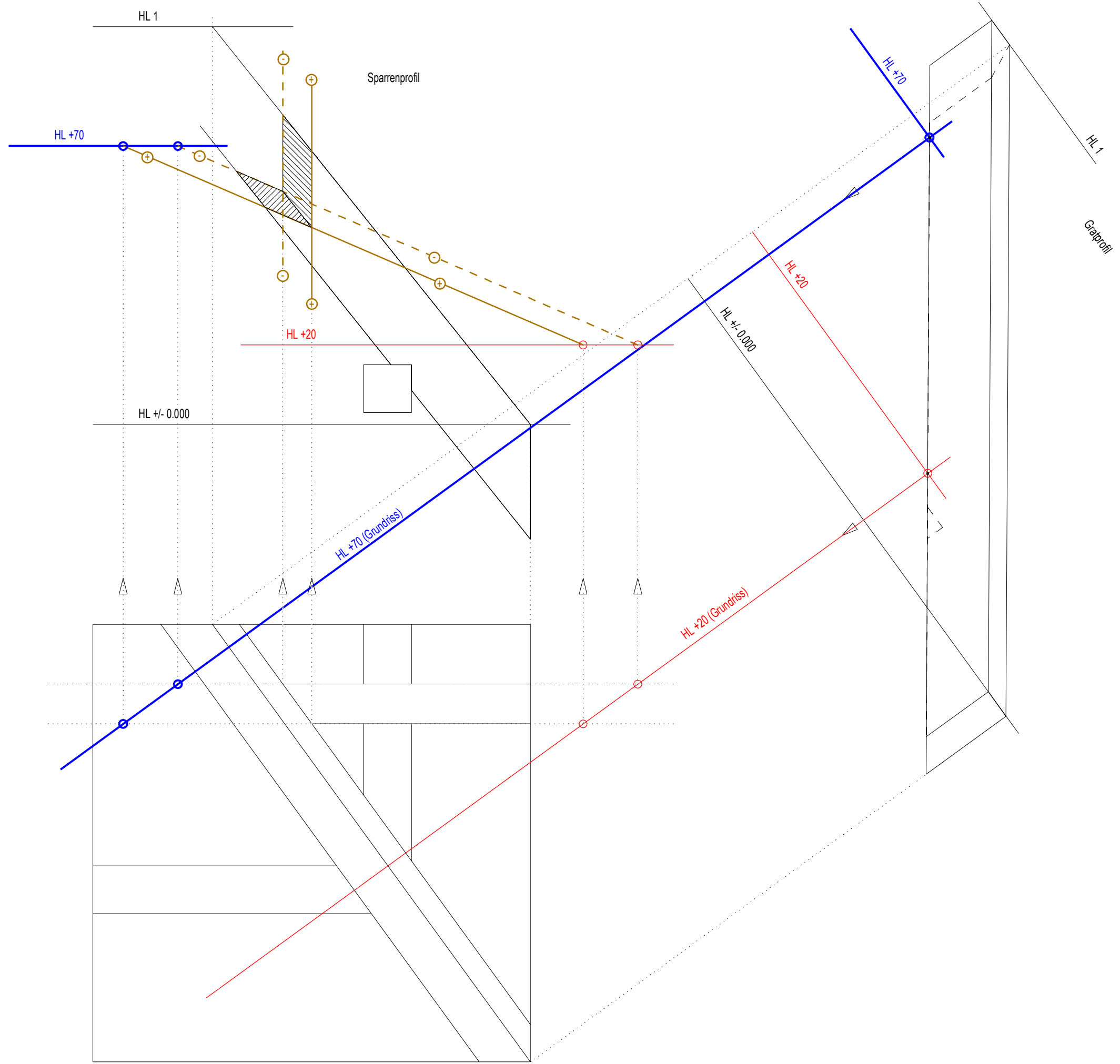
Grundriss
