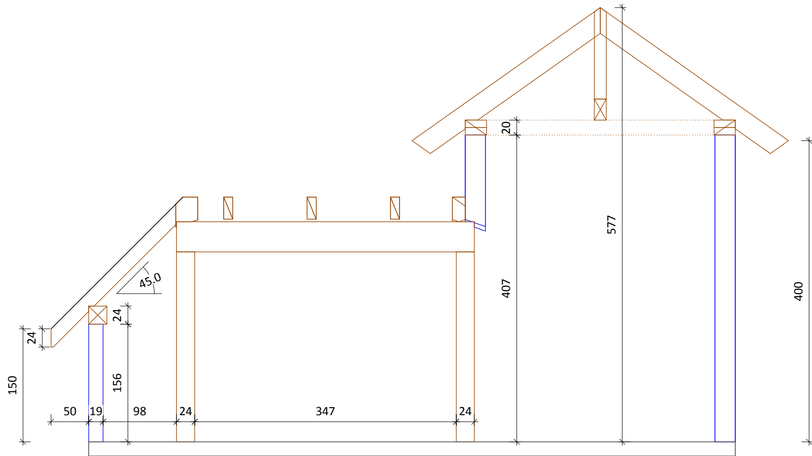
Schnitt A-A
