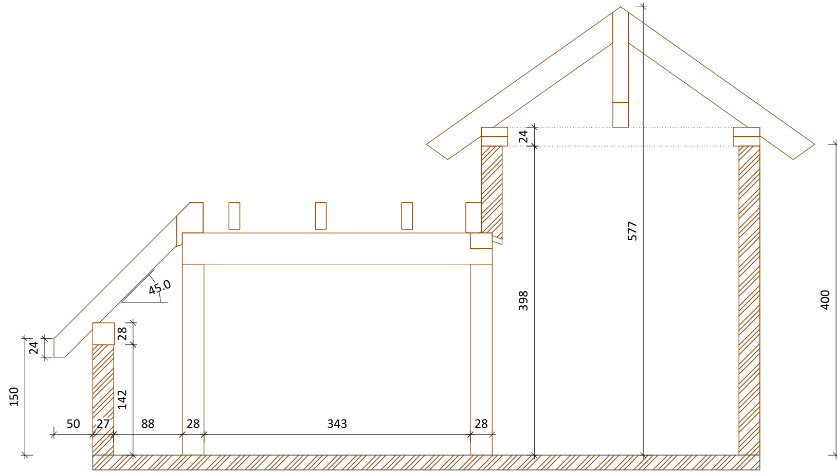
Schnitt A-A
