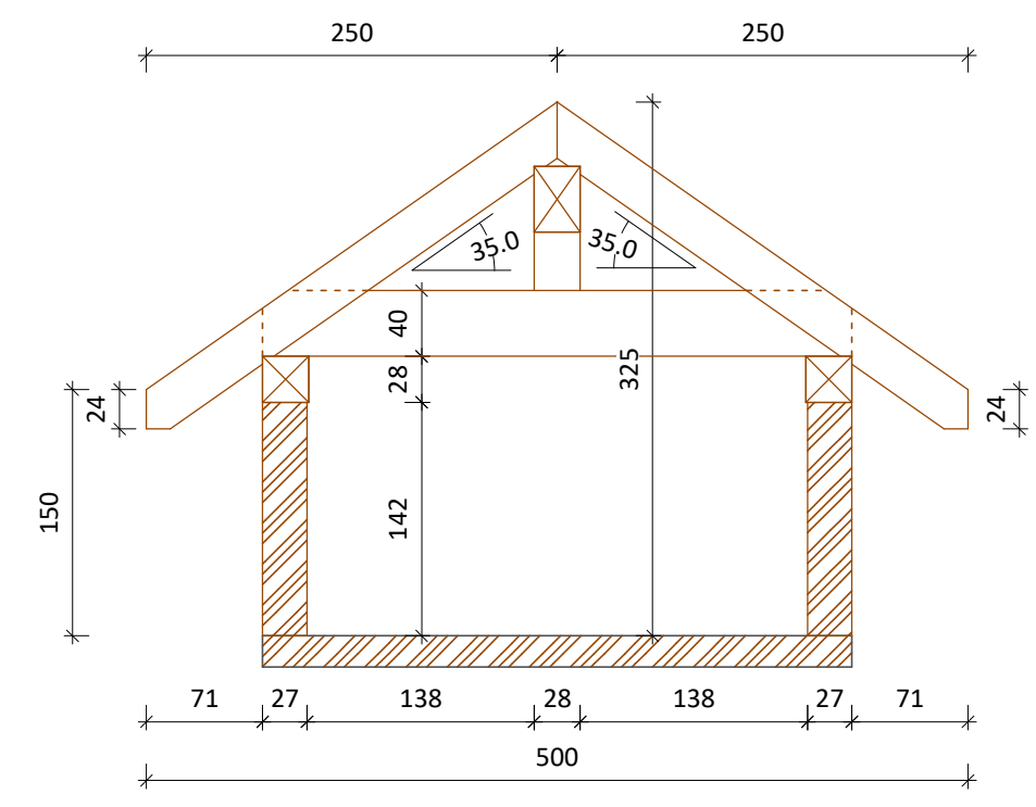
Schnitt B-B
