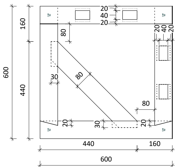
Grundriss unterer Rahmen
