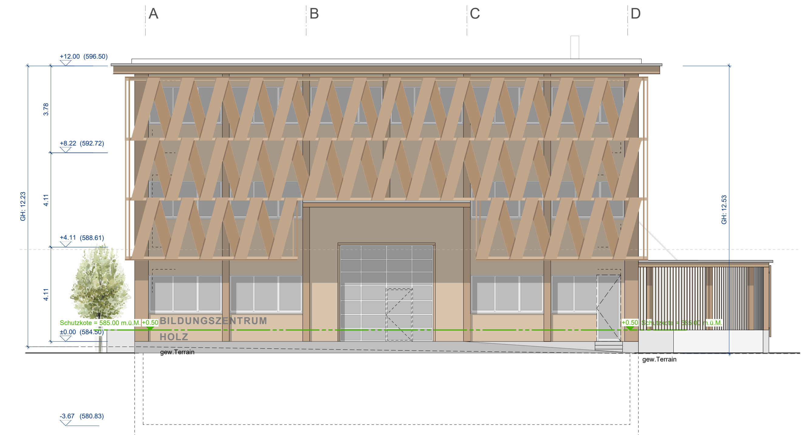
Ostfassade
