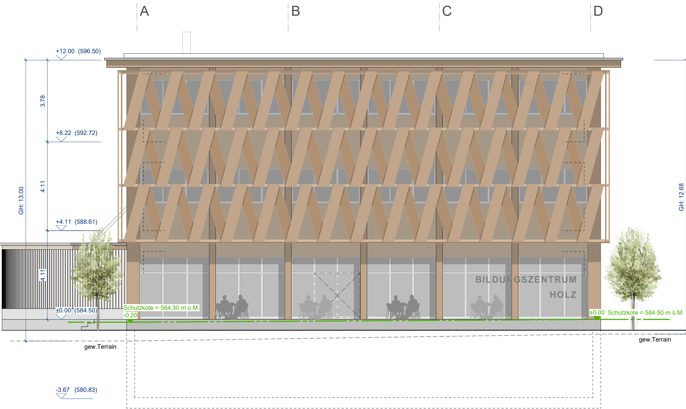
Westfassade
